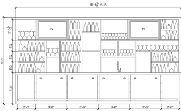
FRONT BAR ELEVATION SCALE: 1/2"=1'-0"
